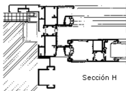
Perfil 3 carriles
