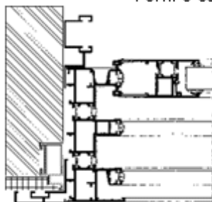
Perfil 3 carriles
